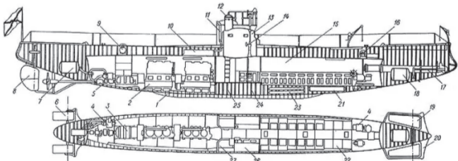
Общее расположение подводной лодки «Минога» 1 — стальной киль; 2 — вальштаг; 3 — стальной аккумуляторный бак; 4 — цитробок; 5 — узелный подшипник; 6 — паровые горизонтальные рули; 7 — паровые дифференциальные цистерны; 8 — вертикальный руль; 9 — горизонтальный бак; 10 — аккумуляторный бак; 11 — шлюзовая заслонка; 12 — рубочный ярус; 13 — боевая рубка; 14 — внутренняя вертикальная труба; 15 — носовое отделение; 16 — паровая вышка; 17 — турбинный аппарат; 18 — носовая дифференциальная цистерна; 19 — носовые горизонтальные рули; 20 — орудийные рубки; 21 — аккумуляторы для торпедной стрельбы; 22 — аккумуляторы; 23 — аккумуляторы для зарядки цистерн; 24 — носовая средняя цистерна; 25 — аккумулятор для обфорта; 27 — топливные цистерны
