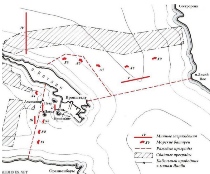
План минной обороны Кронштадта
